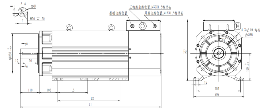
26系列电机尺寸安装图
