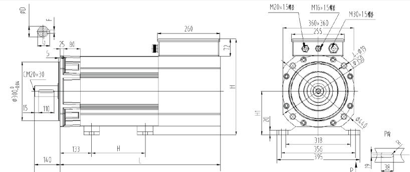
36系列电机尺寸安装图
