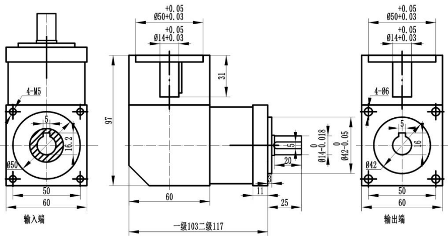
尺寸图 SIZE DIAGRAM
