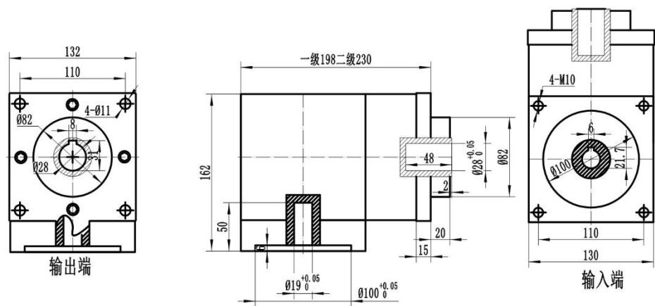
尺寸图 SIZE DIAGRAM
