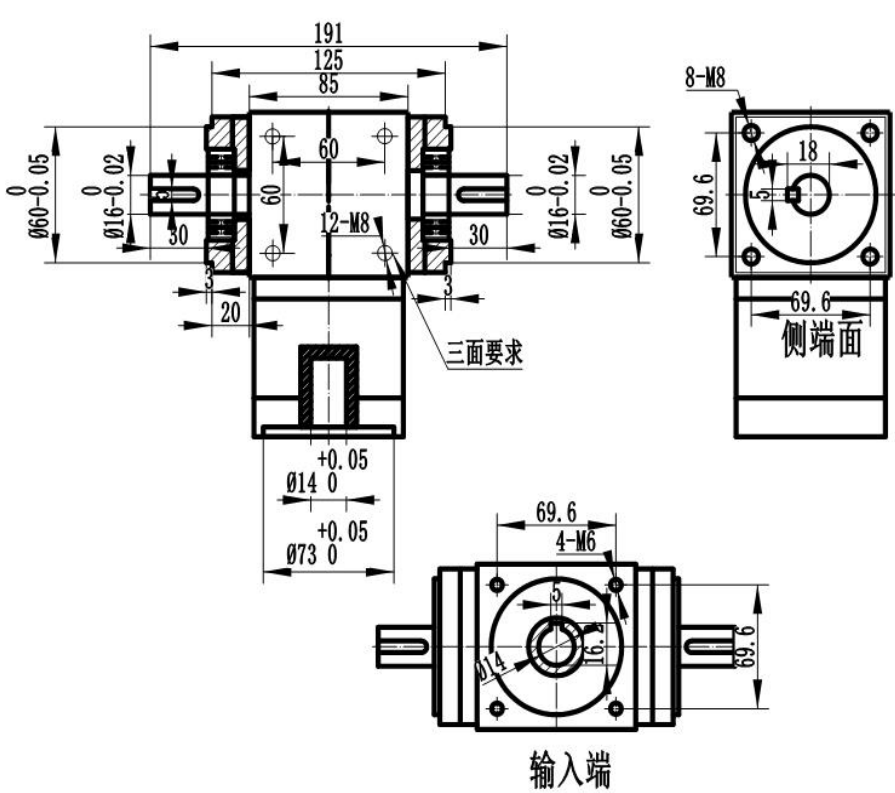
尺寸图 SIZE DIAGRAM
