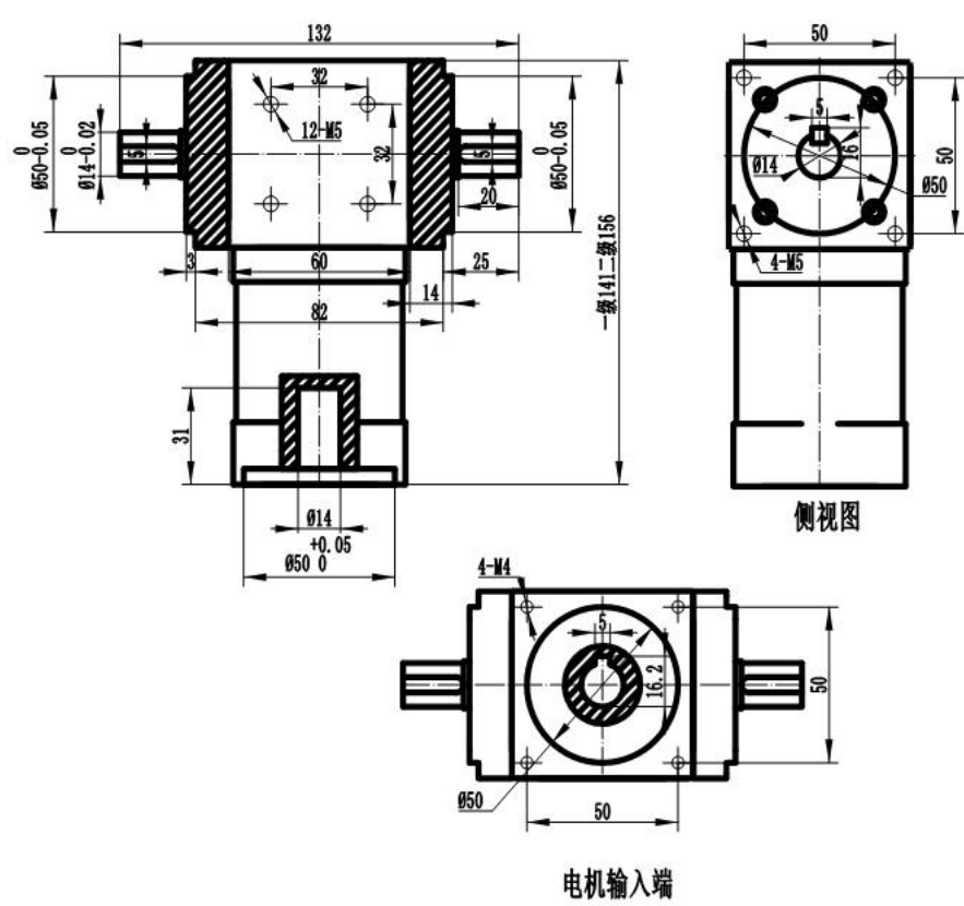
尺寸图 SIZE DIAGRAM
