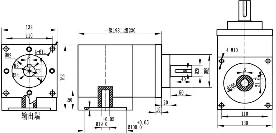
尺寸图 SIZE DIAGRAM
