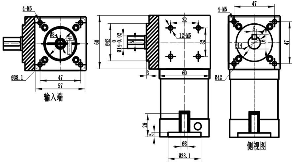
尺寸图 SIZE DIAGRAM
