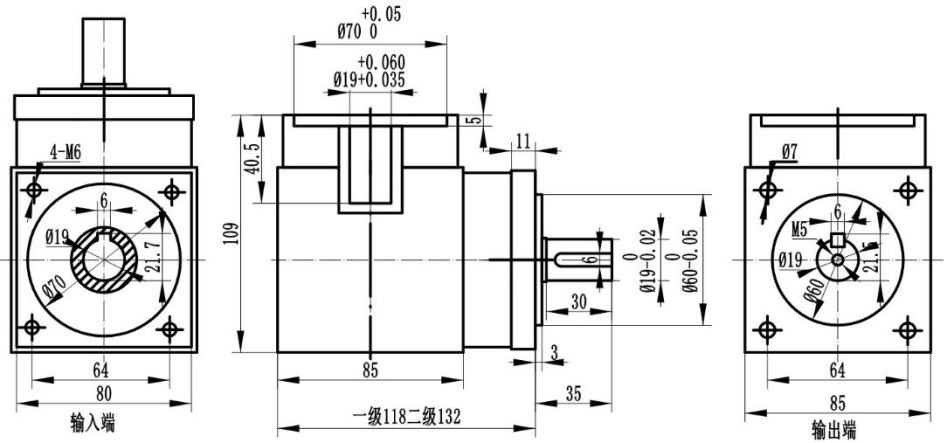
尺寸图 SIZE DIAGRAM
