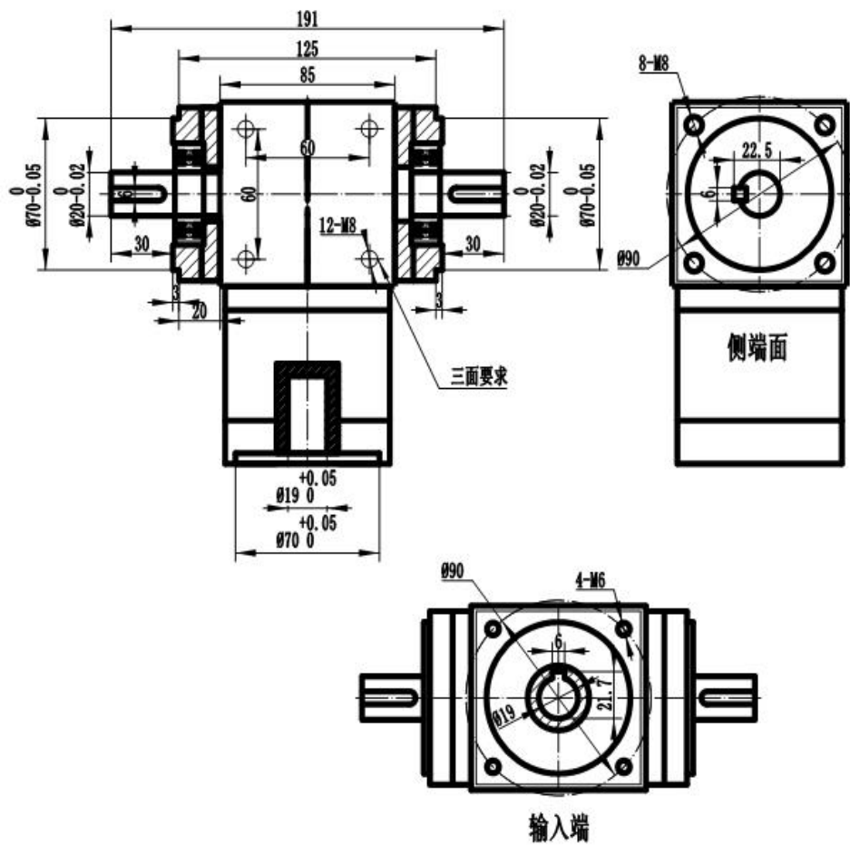
尺寸图 SIZE DIAGRAM
